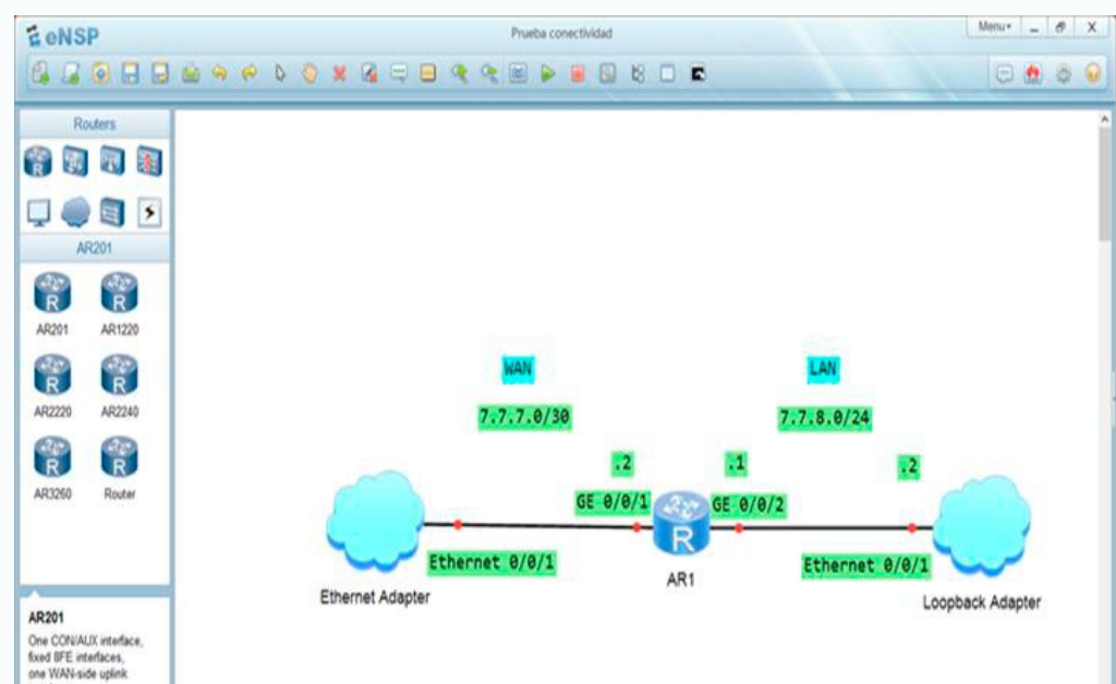
Fig. 2. Topología de red en eNSP
