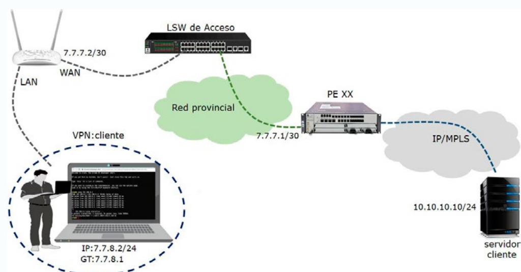
Fig. 1. Arquitectura de red tradicional
