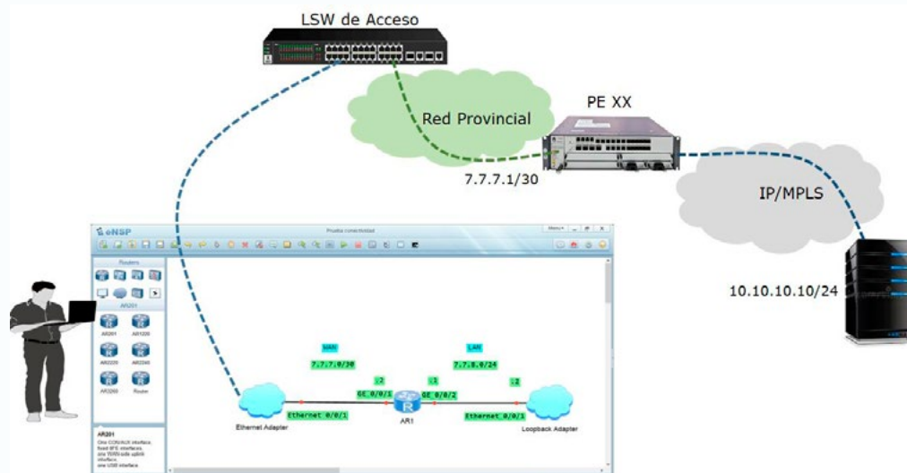
Fig. 3. Arquitectura de red basada en eNSP.
