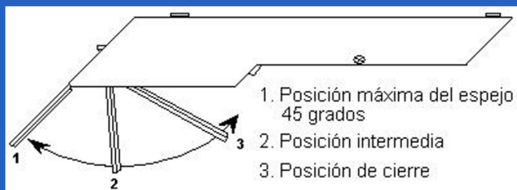
Fig. 2. Diferentes ángulos de visualización del espejo explorador.
