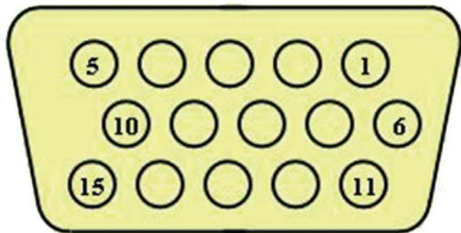
Fig.4. Conector VGA. (Hembra)
